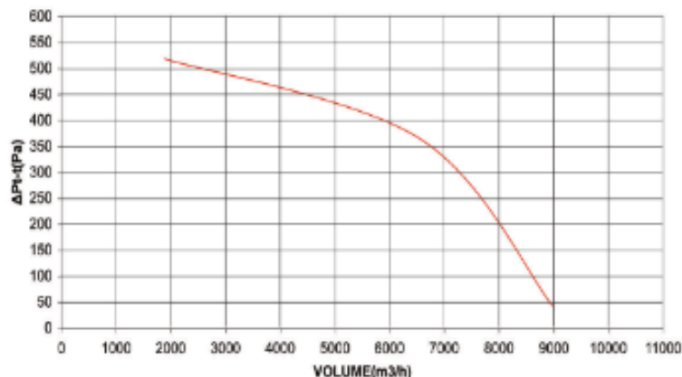
Φ350-3.0HP-1450RPM
